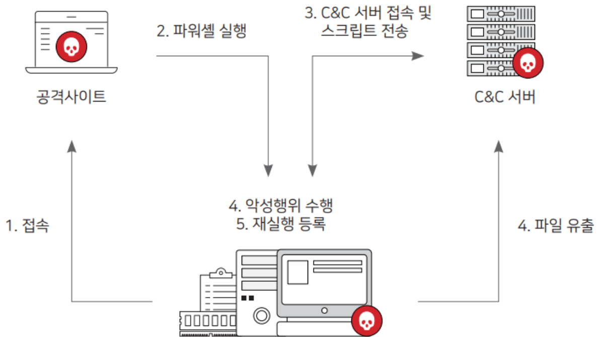
[그림 4. 일반적인 파일리스(Fileless) 공격 흐름]
